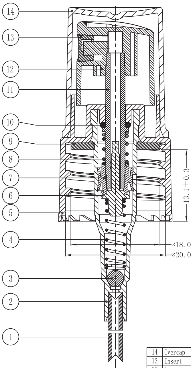
Section A-A
